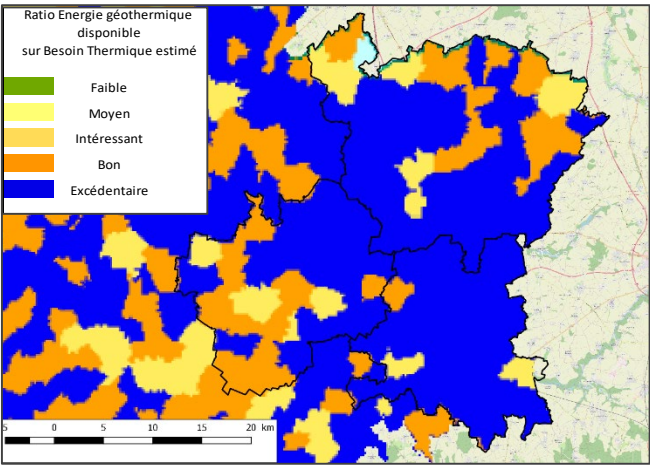
Carte des zones favorables pour la géothermie (Source : BRGM)
